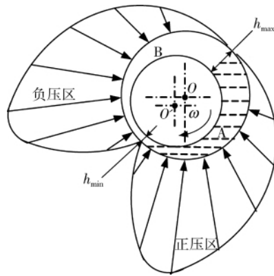
图 1 滑动轴承工作原理图
