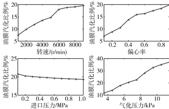
图 7 油膜气化比例影响因素分析
