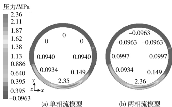
图 5 滑动轴承油膜压强分布
