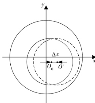
图 4 滑动轴承动力特性求解模型
