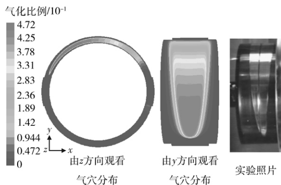
图 6 滑动轴承气液两相分布
