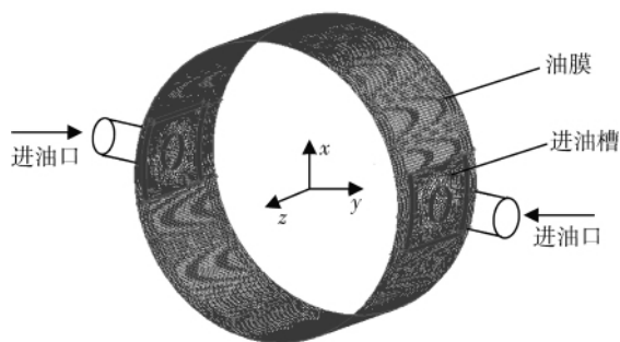
图 3 滑动轴承网格结构图
